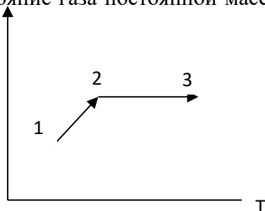
Рисунок 1 – Зависимость объема газа от термодинамической температуры
